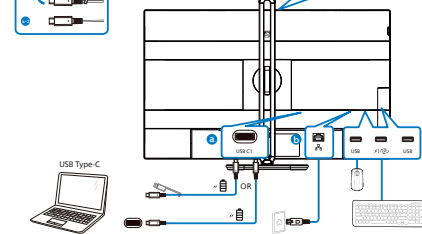
USB hub (USB A-C)
