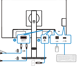
USB docking (USB C-C)
