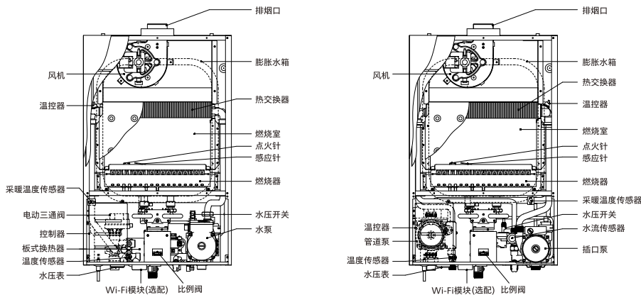
L1P36-AWH7334/93(B32C1G)、L1P40-AWH7335/93(B36C2G)内部机构图
