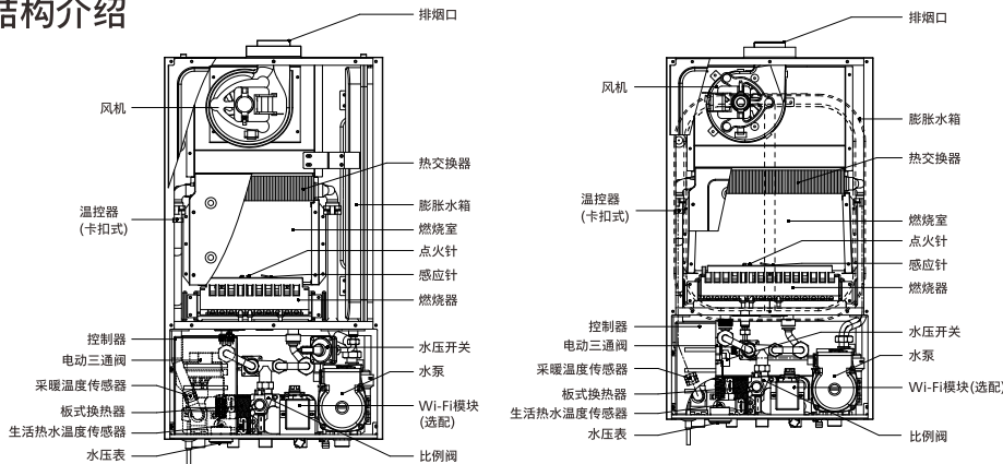
L1P24-AWH7331/93(B20C1G) 内部结构图
