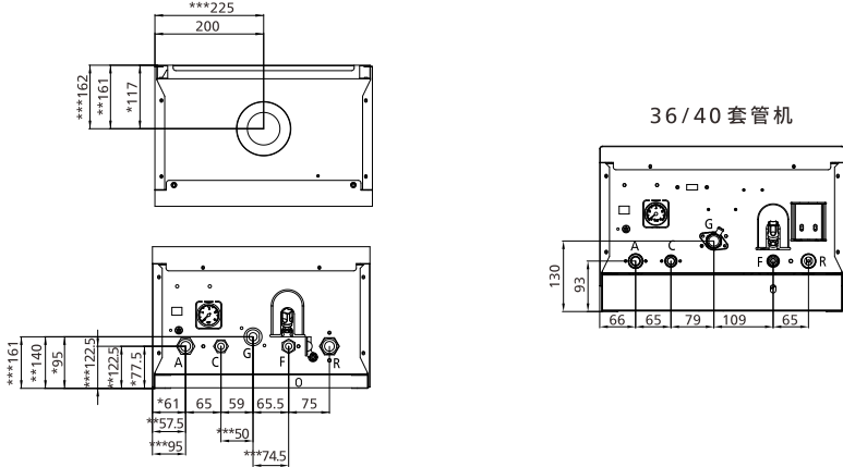
管路接口示意图
