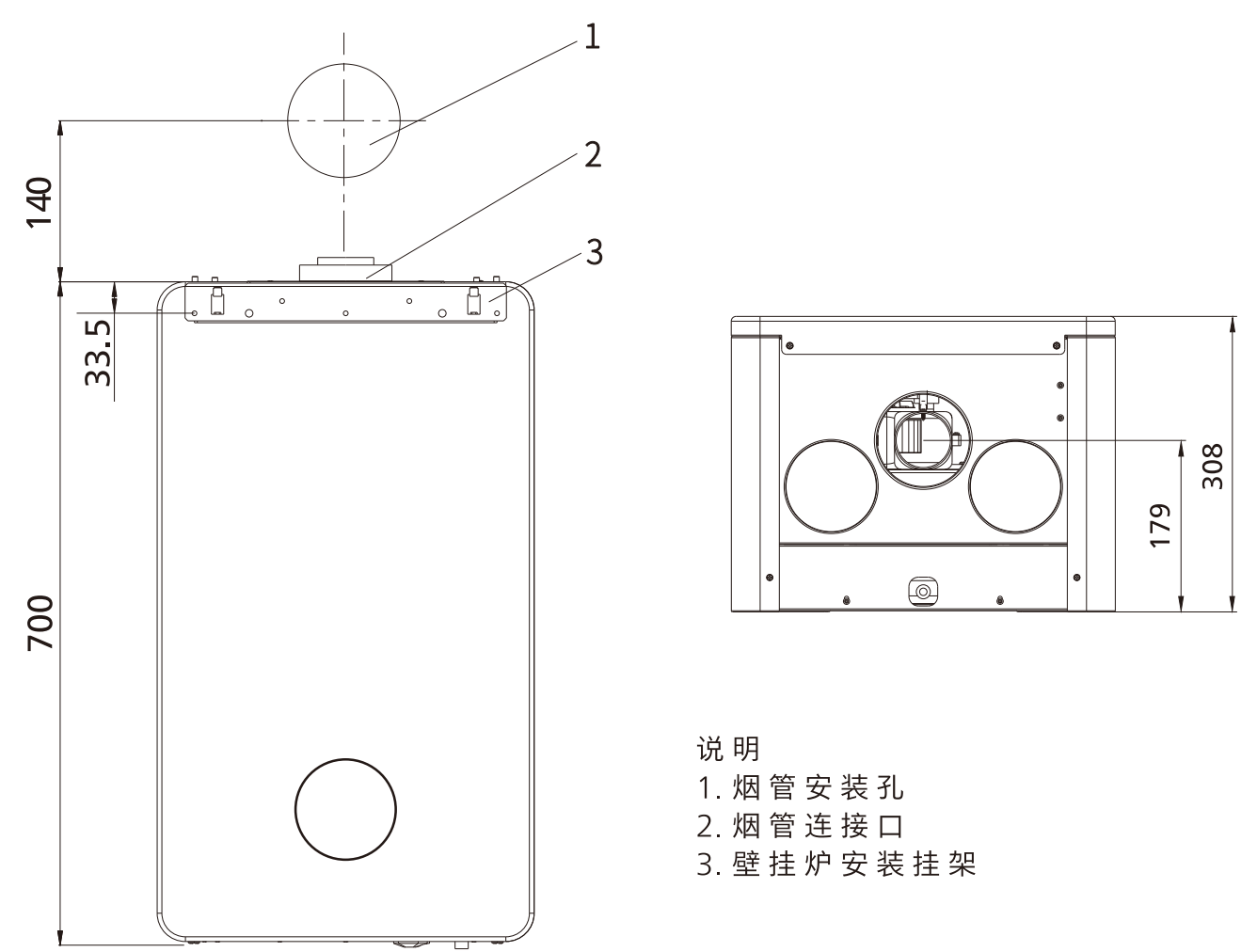
■ 燃气采暖热水炉烟管安装尺寸图
