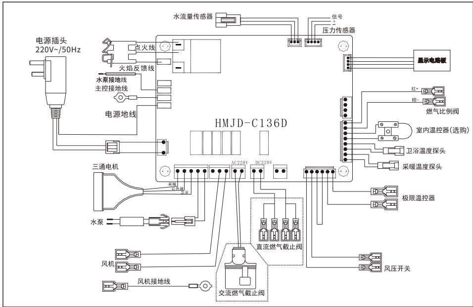
配线图
