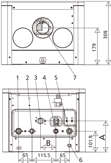
管路接口示意图
