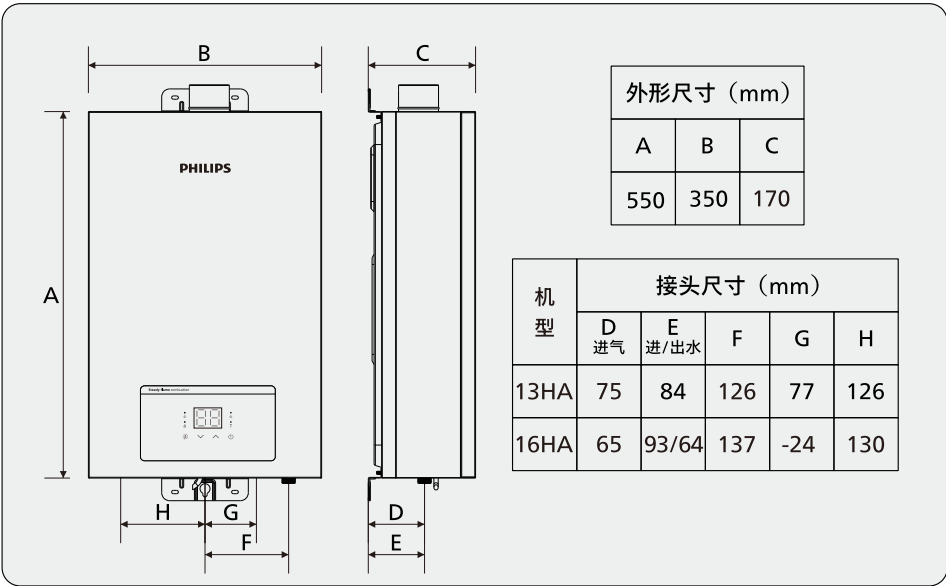
外观结构、部件名称及产品尺寸
