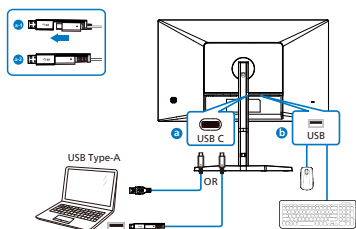
USB A-C
