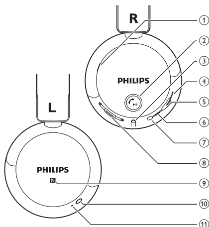
① Micro USB 充電スロット
