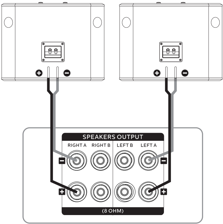
功率放大器
