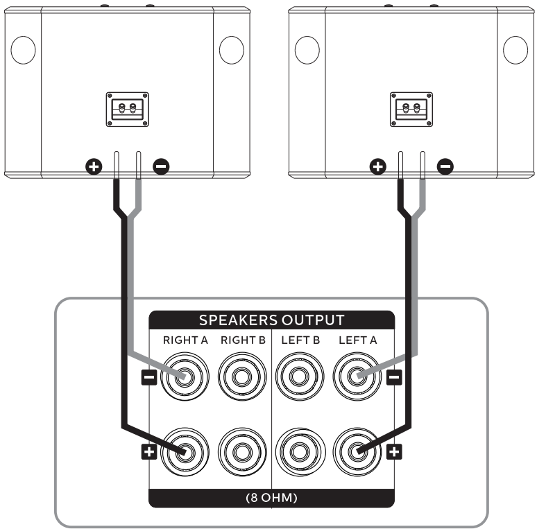
功率放大器
