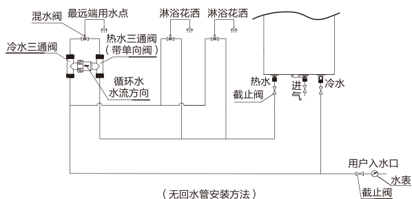
(无回水管安装方法)
