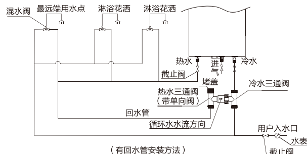
(有回水管安装方法)
