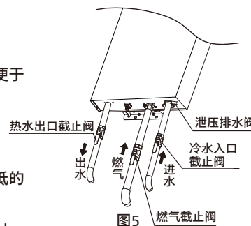
图5 燃气截止阀
