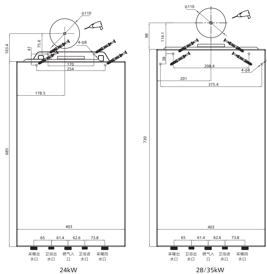
■ 燃气采暖热水炉烟管安装尺寸图
