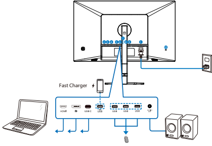
USB C-C
