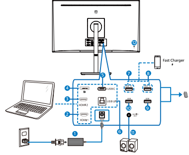
USB C-C
