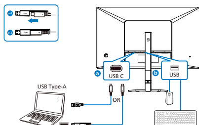
USB A-C
