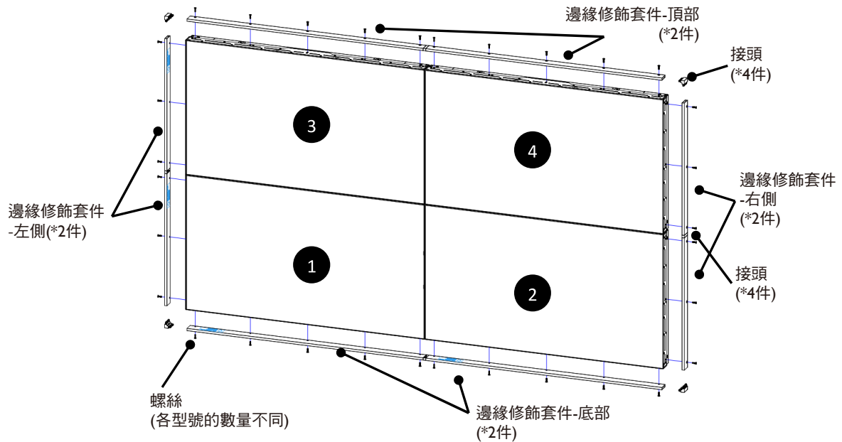
安裝適用於 2x2 顯示器配置的邊緣修飾套件
