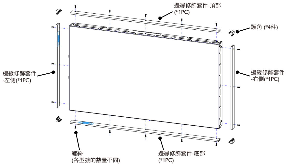
安裝適用於 1x1 顯示器配置的邊緣修飾套件
