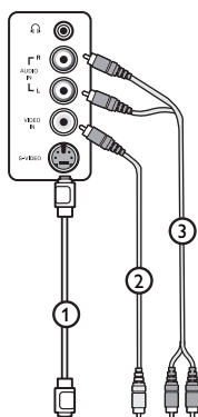
Złącza z boku telewizora
