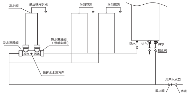
(无回水管安装方法)
