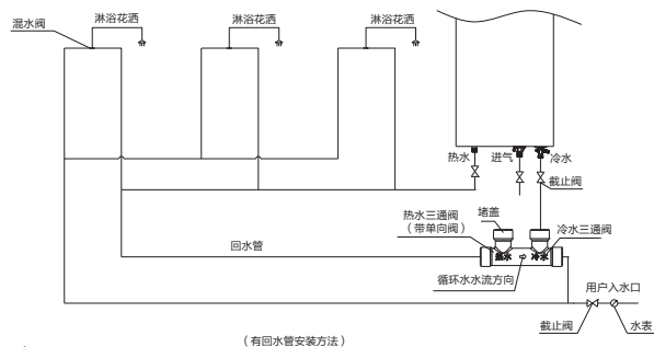
(有回水管安装方法)
