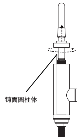
泄压复位示意图
